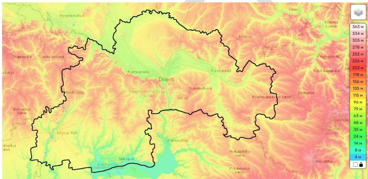
Рисунок 3: Рельєф Дніпропетровської області
